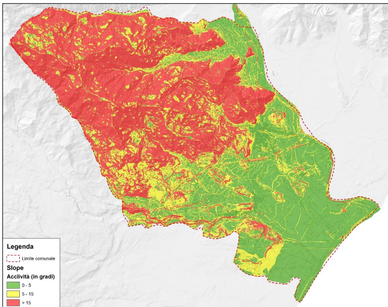
Figura 3: Carta delle pendenze per il territorio comunale di Calatabiano.
