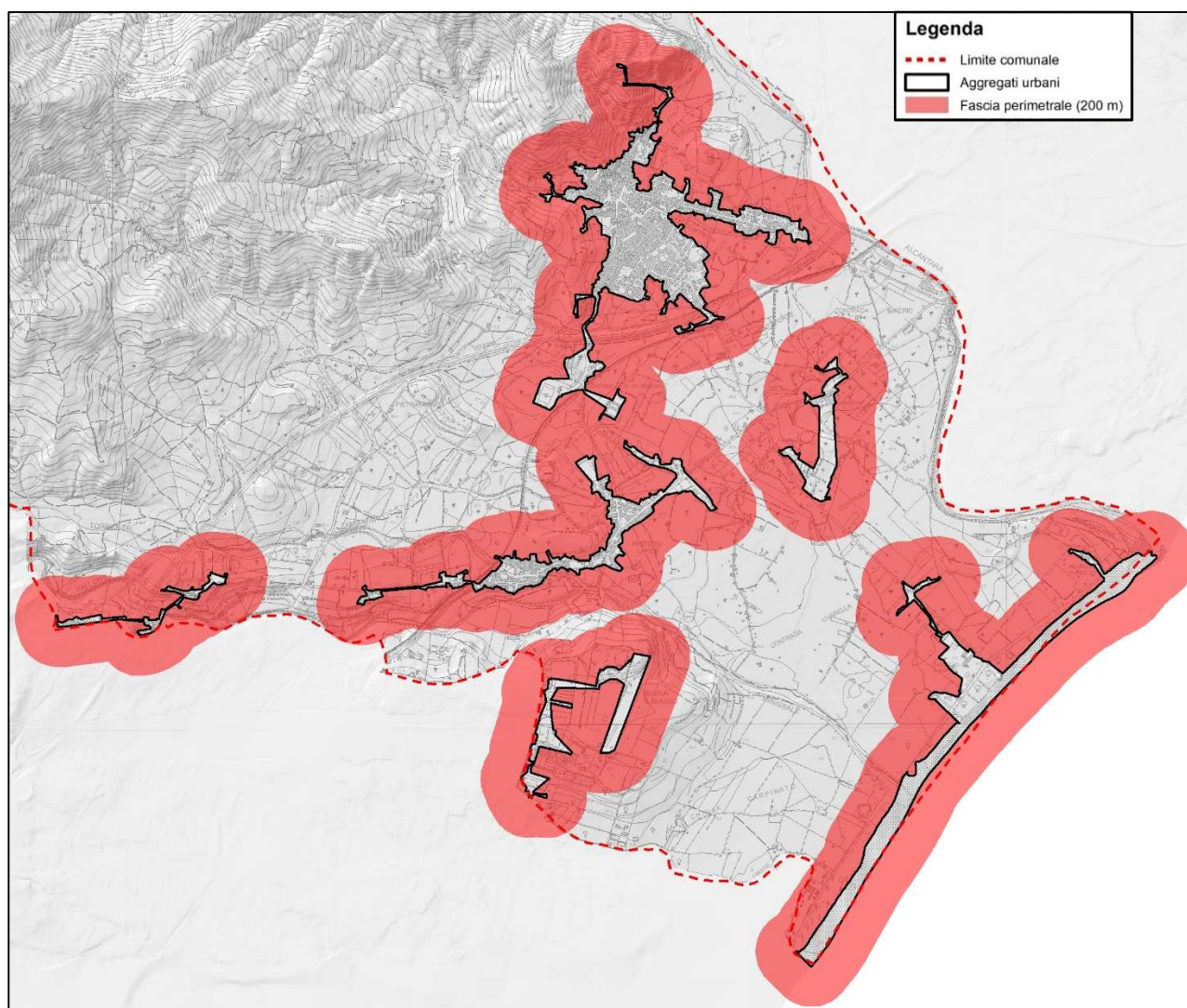
Figura 1: Aree antropizzate (linea nera) e fascia perimetrale (area rossa) di 200 metri utilizzata ai fini della valutazione della pericolosità agli incendi di interfaccia. Base cartografica: Carta Tecnica Regionale (CTR) 2012, i limiti comunali sono rappresentati con la linea rossa tratteggiata.
