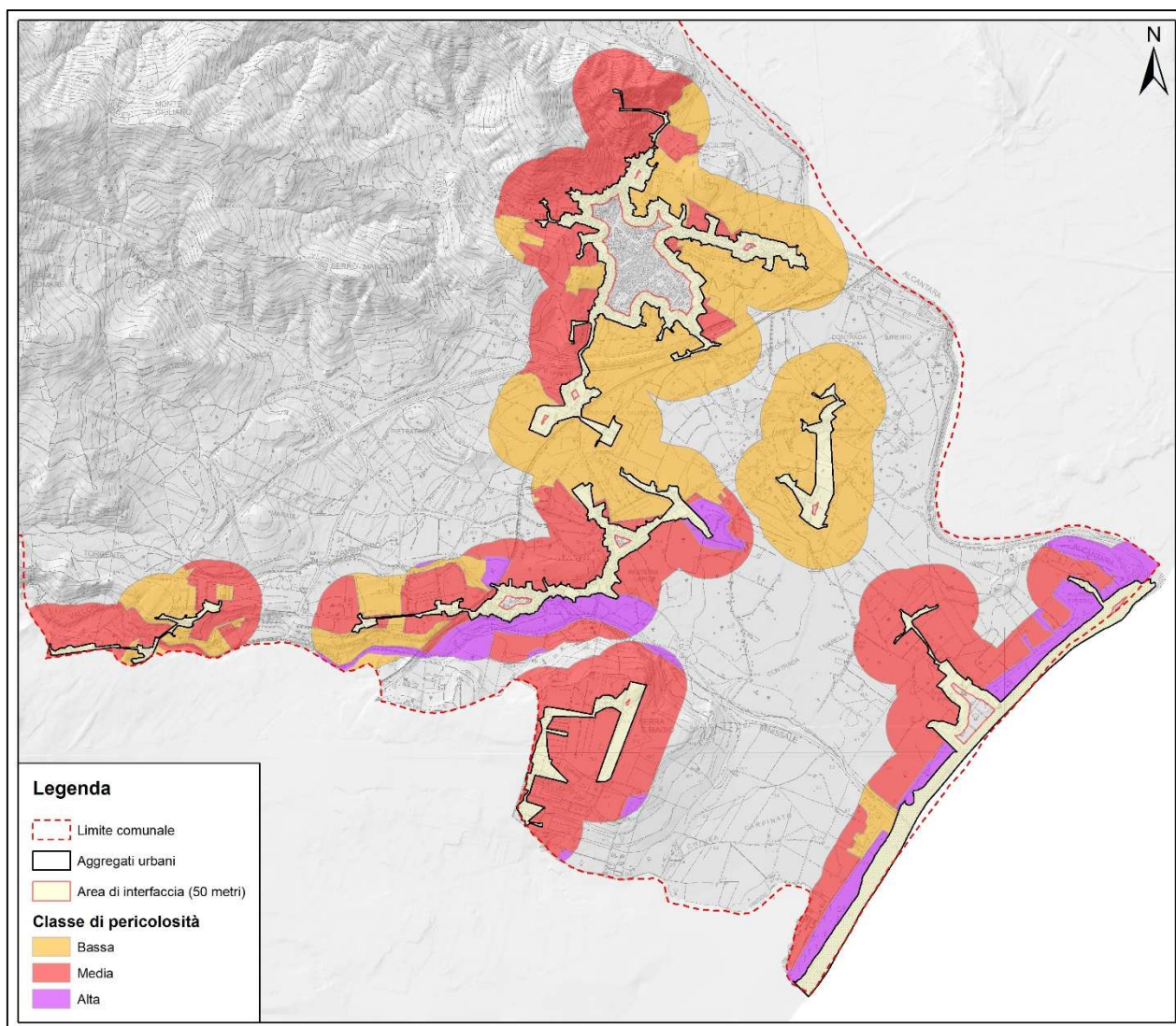
Figura 5: Carta della pericolosità agli incendi di interfaccia. Con la linea continua nera è rappresentata l'area antropizzata. Base cartografica: CTR 2012/2013, i limiti comunali sono rappresentati con la linea rossa tratteggiata.
