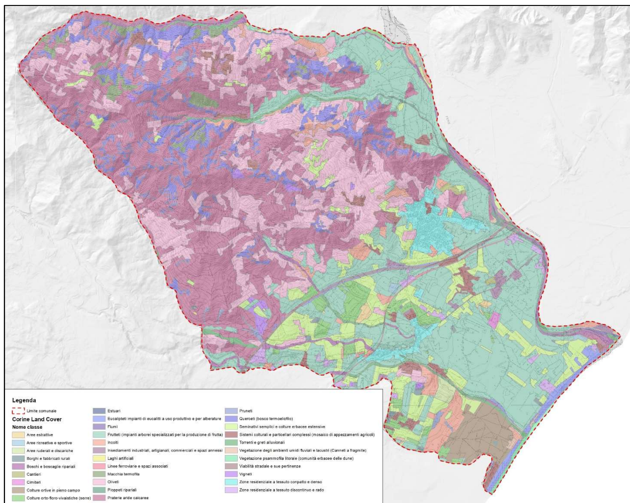
Figura 2: Carta Corinne Land Cover (copertura ed uso del suolo) per il territorio comunale di Calatabiano.
