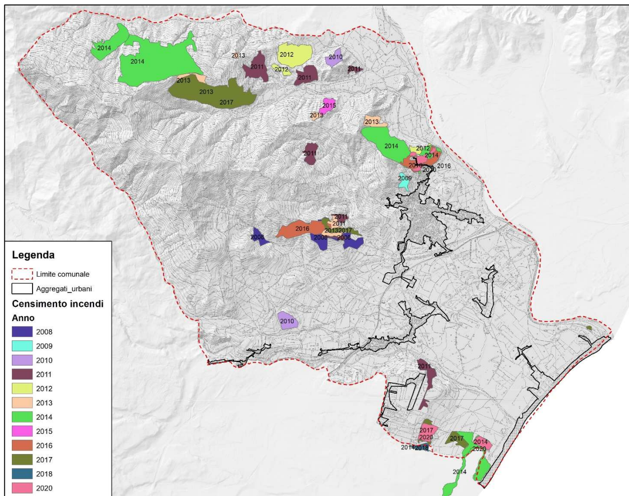
Figura 4: Ubicazione incendi pregressi (Catasto incendi).
