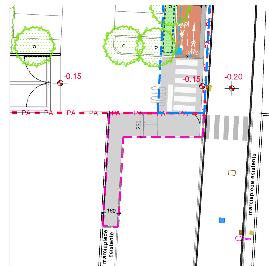
LEGENDA PERIMETRO PIANO DI LOTTIZZAZIONE VERDE PUBBLICO PISTA CICLO-PEDONALE IN PROGETTO AREA A PARCHEGGIO AREA A STANDARD IN CESSIONE AREE ESTERNE AL P.L. DA RIQUALIFICARE QUOTE IN PROGETTO RETE FOGNATURE ACQUE BIANCHE Caditoia stradale esistente Linea tombinatura esistente Pozzo perdente esistente RETE PUBBLICA ILLUMINAZIONE Illuminazione pubblica esistente Rete Illuminazione Pubblica Ø125 tubo corrugato (in progetto) Anello 40x40 con chiusura in ghisa sferoidale (in progetto) Pali fino a 8m, sbraccio fino a 2m e proiettore a LED. (in progetto) Pozzetto-pilino per palo Pubbl. Illuminazione 70x100x100 con tasca quadrata da 40x40 interna e tasca circolare Ø27 con chiusura in ghisa sferoidale C250 luce 44x44 (in progetto) RETE IDRICA Rete idrica Ø50 / Ø32 PEAD (in progetto) Pozzetto per collocamento elettrovalvole (in progetto)
