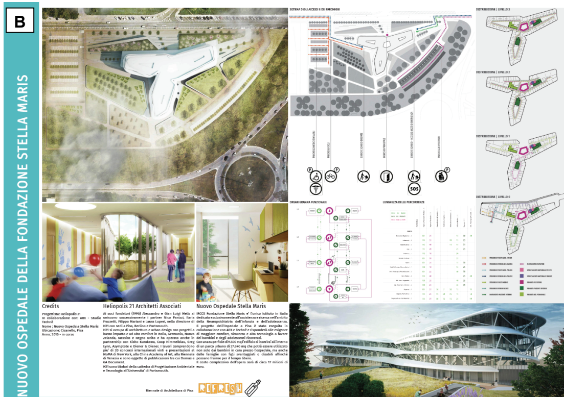
Figura 31 – “Stella Maris”: lay-out dell’area e schema di progetto
