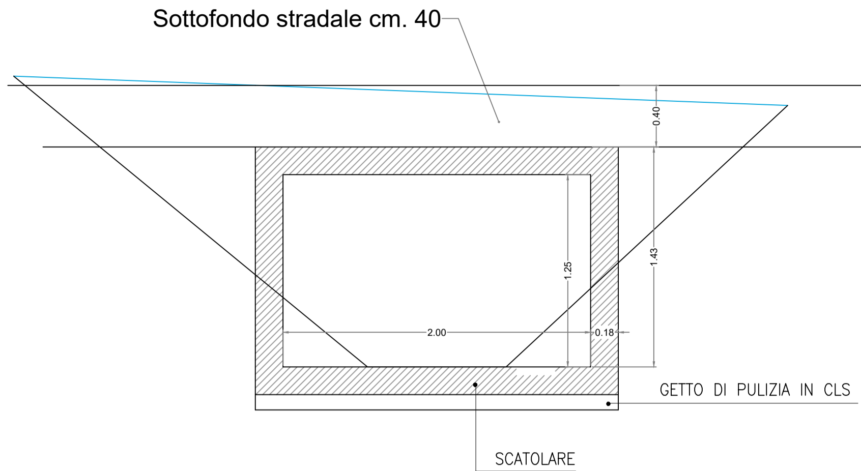
PARTICOLARE SCATOLARE A SEZIONE RETTANGOLARE, PER FOSSO scala: 1:25
