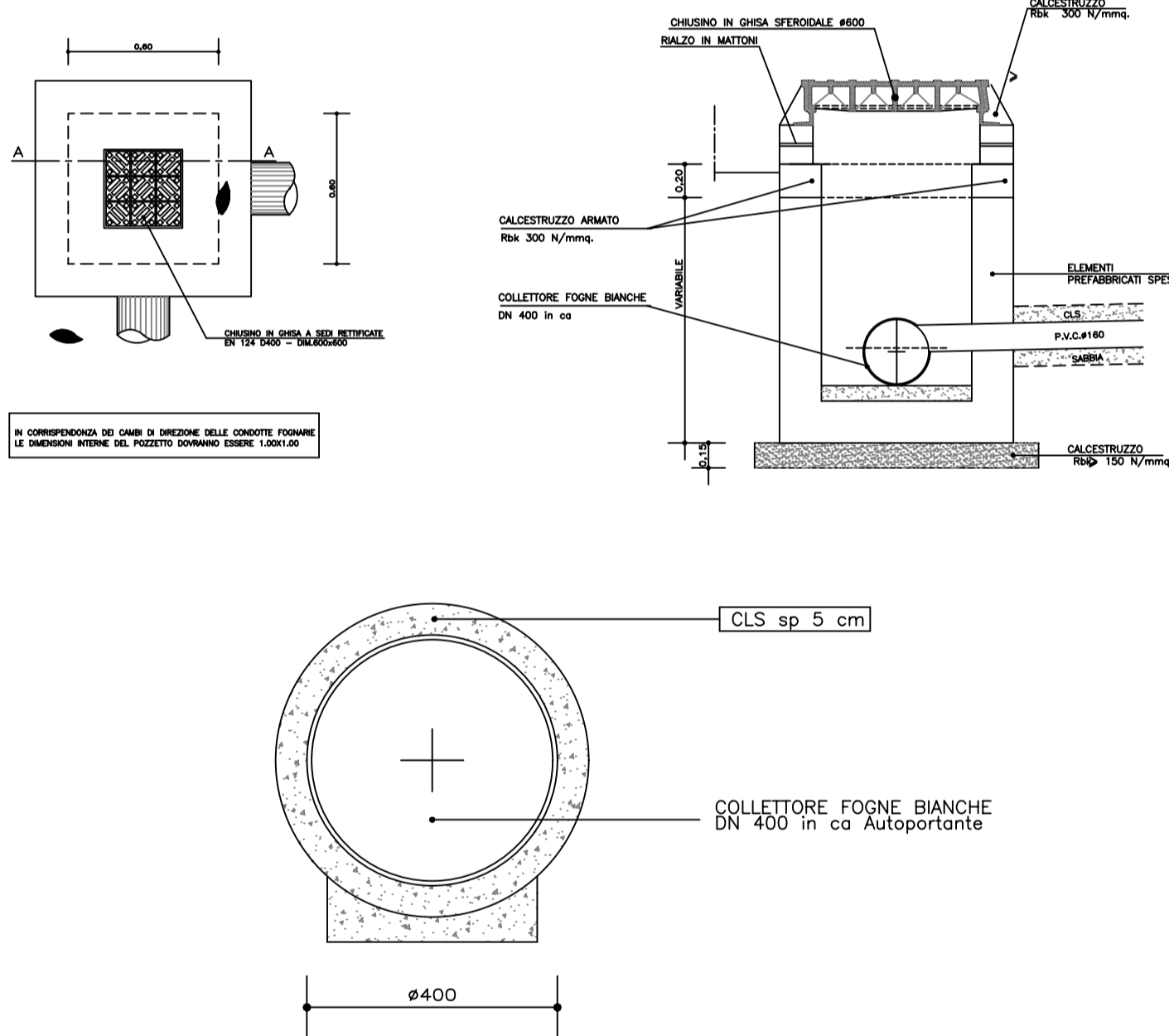
PARTICOLARE POZZETTO D'ISPEZIONE FOGNATURA ACQUE BIANCHE scala: 1:25
