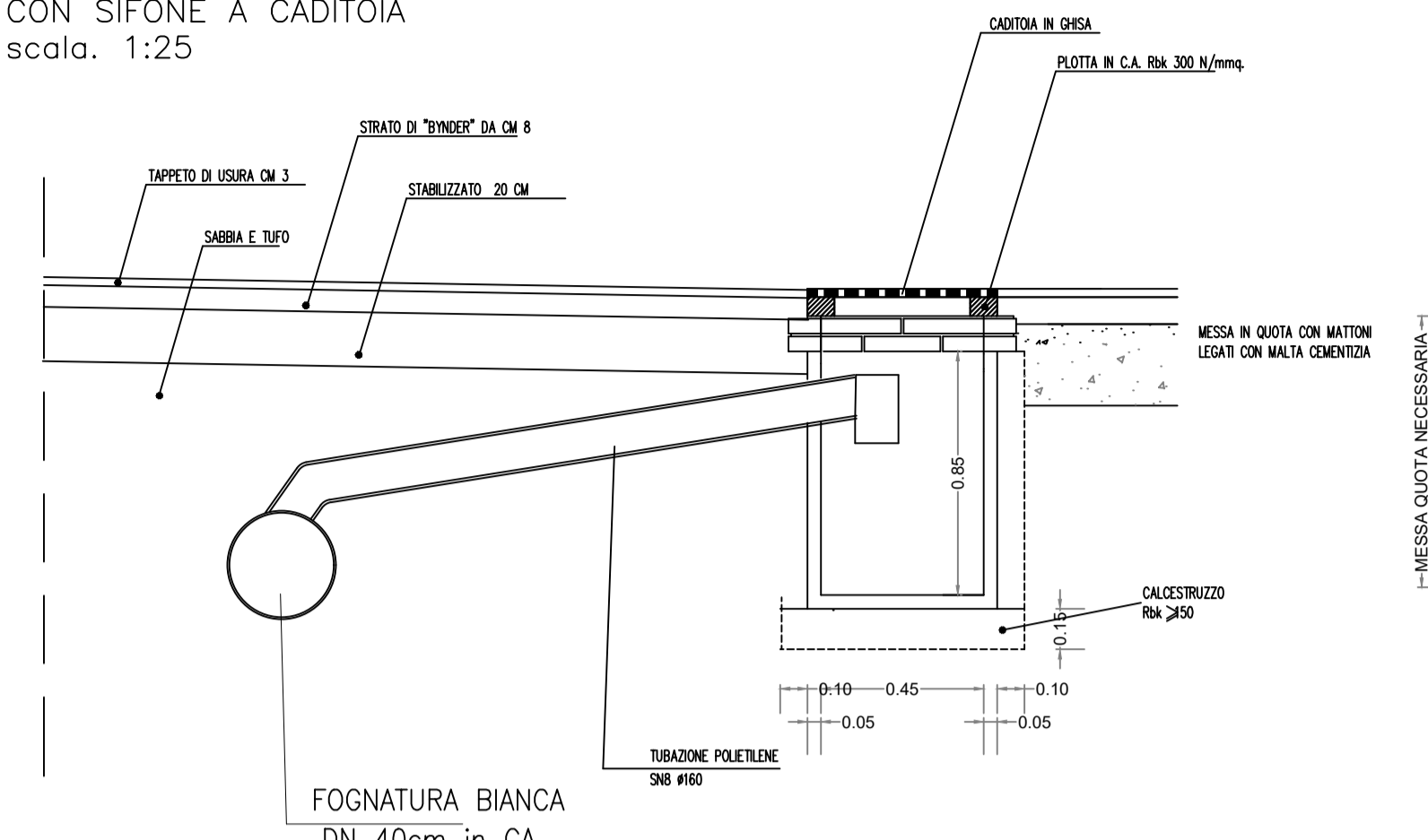
PARTICOLARE POZZETTO CON SIFONE A CADITOIA scala: 1:25
