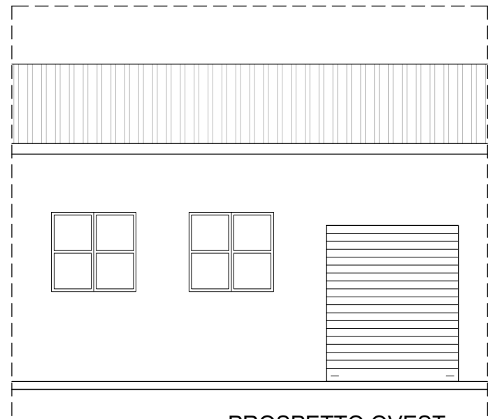
PROSPETTO OVEST
