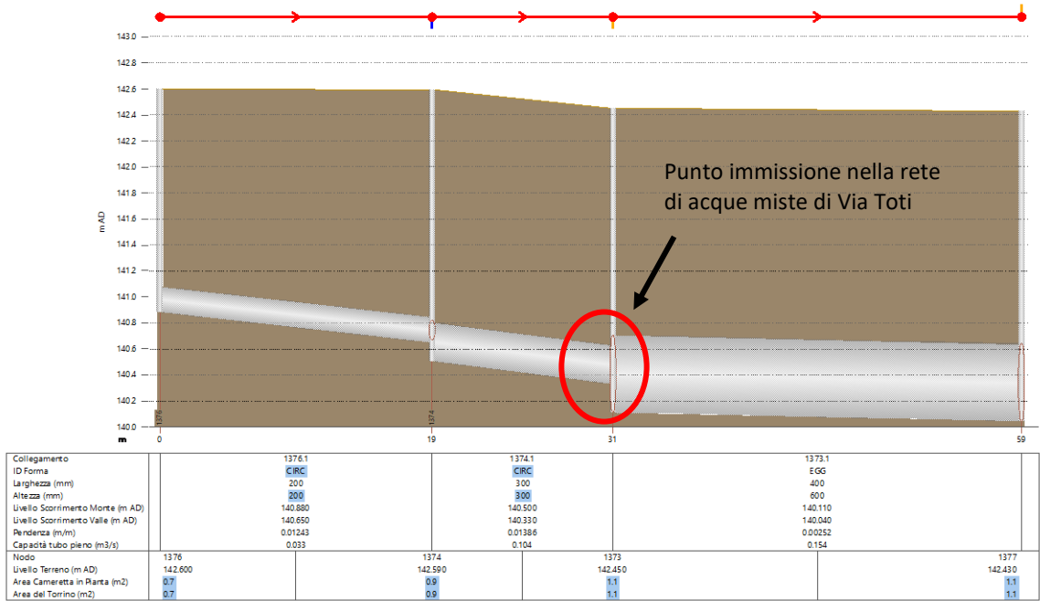
Figura 5 – Profilo condotta acque bianche stato di fatto (parcheggio ovest)
