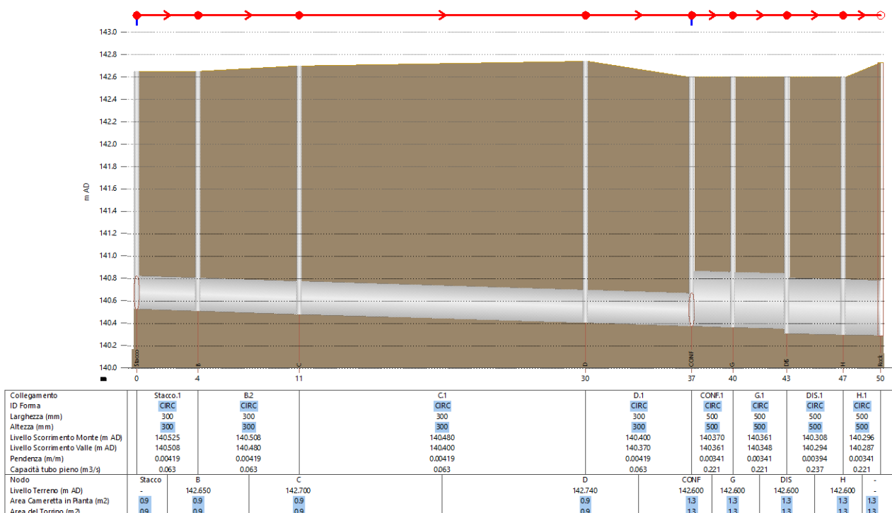
Figura 7 – Profilo nuova rete acque meteoriche dal parcheggio est
