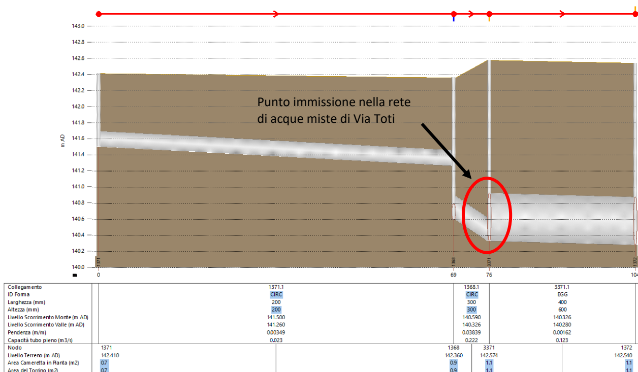
Figura 6 – Profilo condotta acque bianche stato di fatto (parcheggio est)
