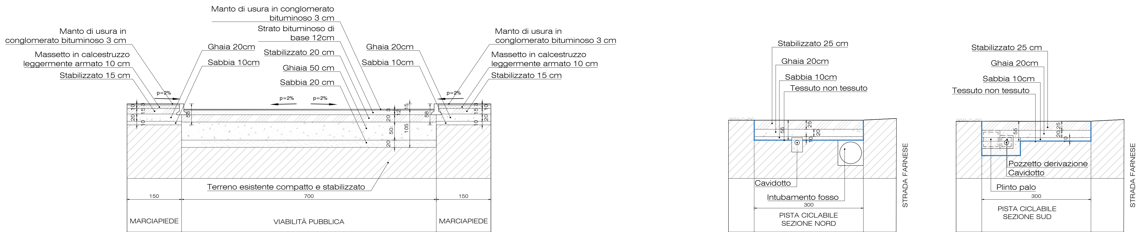
SEZIONE 2-2
