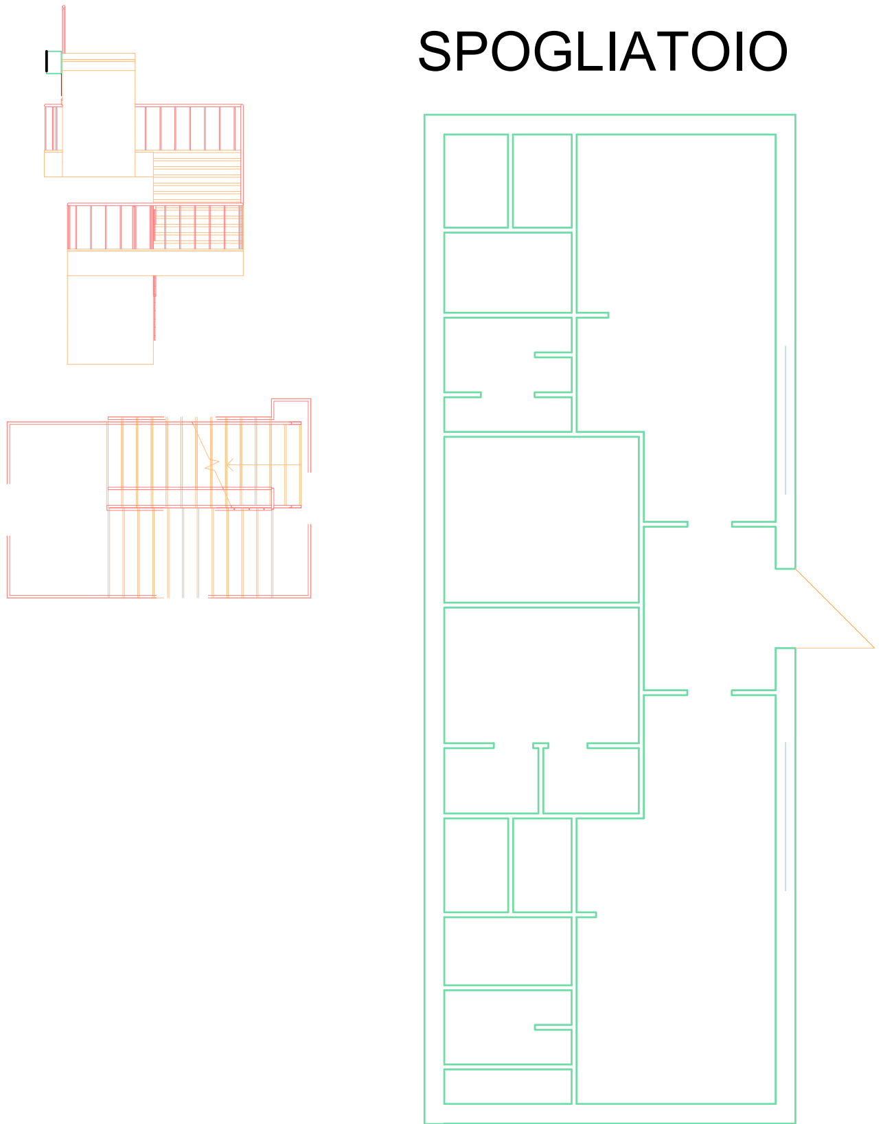
PIANTA SPOGLIATOIO ESISTENTE
