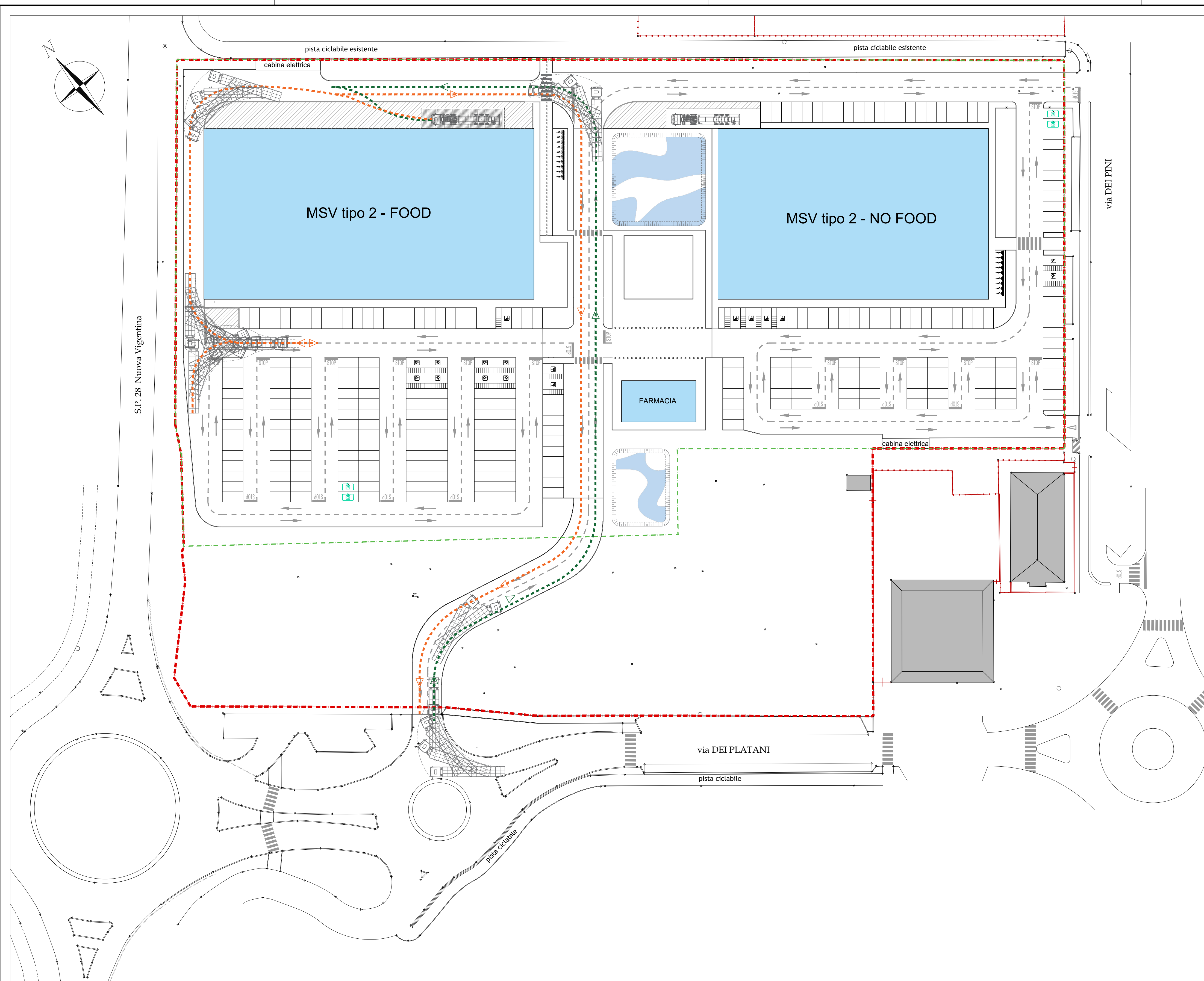
VIABILITA' INTERNA PER MEZZI PESANTI - EDIFICIO TIPO 2 MSV FOOD scala 1:500
