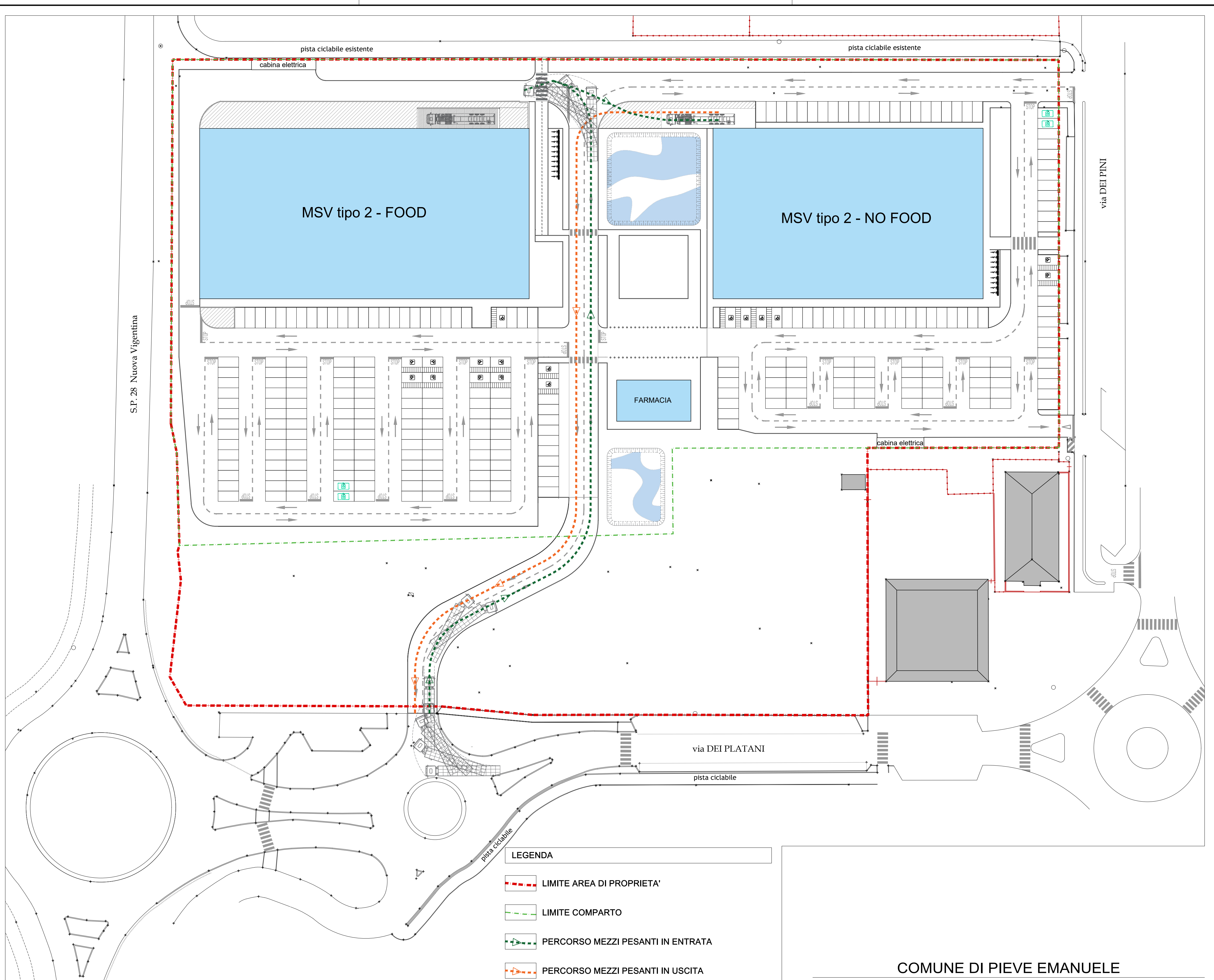
VIABILITA' INTERNA PER MEZZI PESANTI - EDIFICIO TIPO 2 MSV NO FOOD scala 1:500
