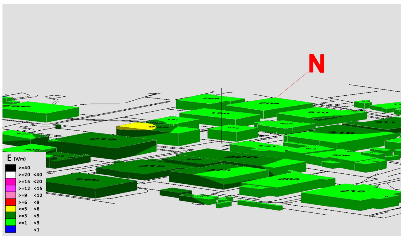
Fig. 35 Impatto elettromagnetico - Zona Area Comunale Via dell'Industria - Vista Laterale 2
