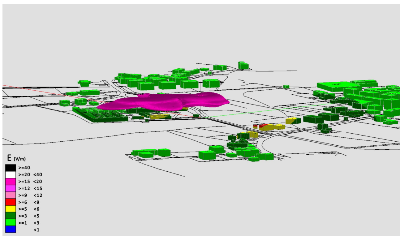
Fig. 14 Impatto elettromagnetico - Zona Cimitero Piove di Sacco 2 - Vista Laterale 1
