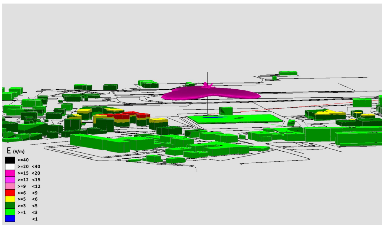
Fig. 4 Impatto elettromagnetico - Zona Area Comunale c/o Stadio - Vista Laterale 1
