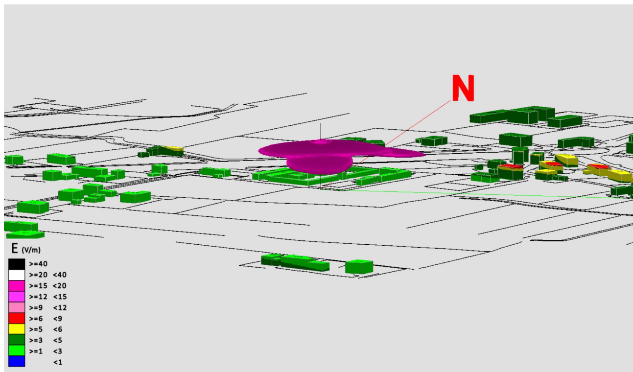
Fig. 39 Impatto elettromagnetico - Zona Cimitero di Corte - Vista Laterale 1
