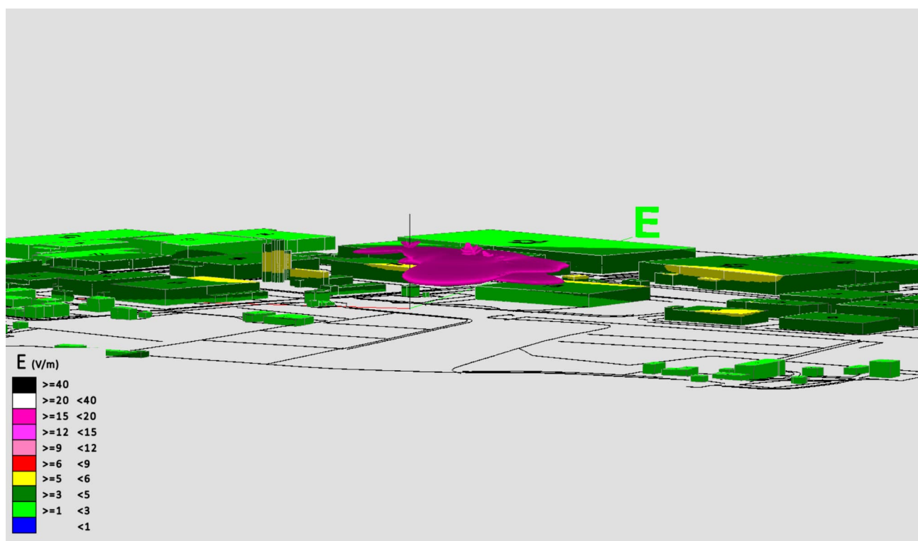
Fig. 19 Impatto elettromagnetico - Zona Area Comunale Via Keplero Nord - Vista Laterale 1
