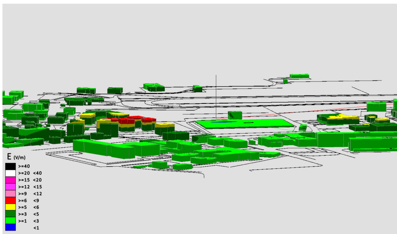
Fig. 5 Impatto elettromagnetico - Zona Area Comunale c/o Stadio - Vista Laterale 2
