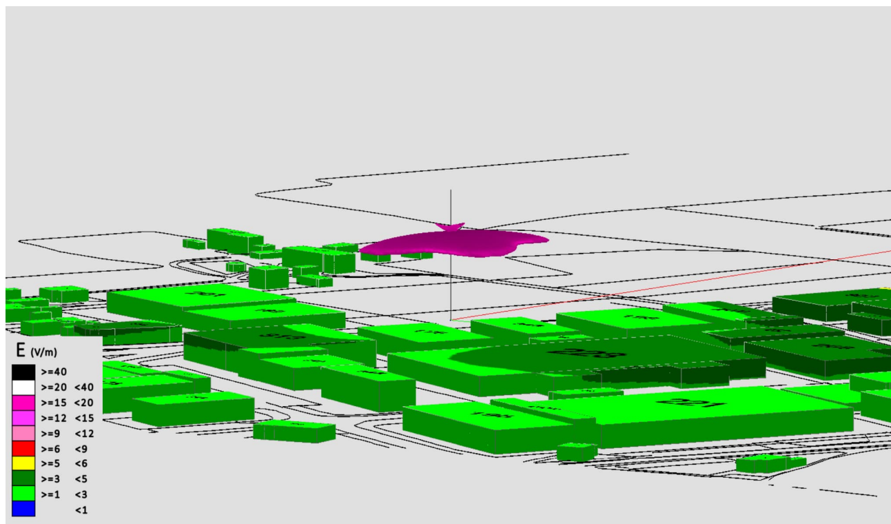
Fig. 24 Impatto elettromagnetico - Zona Area Comunale Via Keplero Sud - Vista Laterale 1
