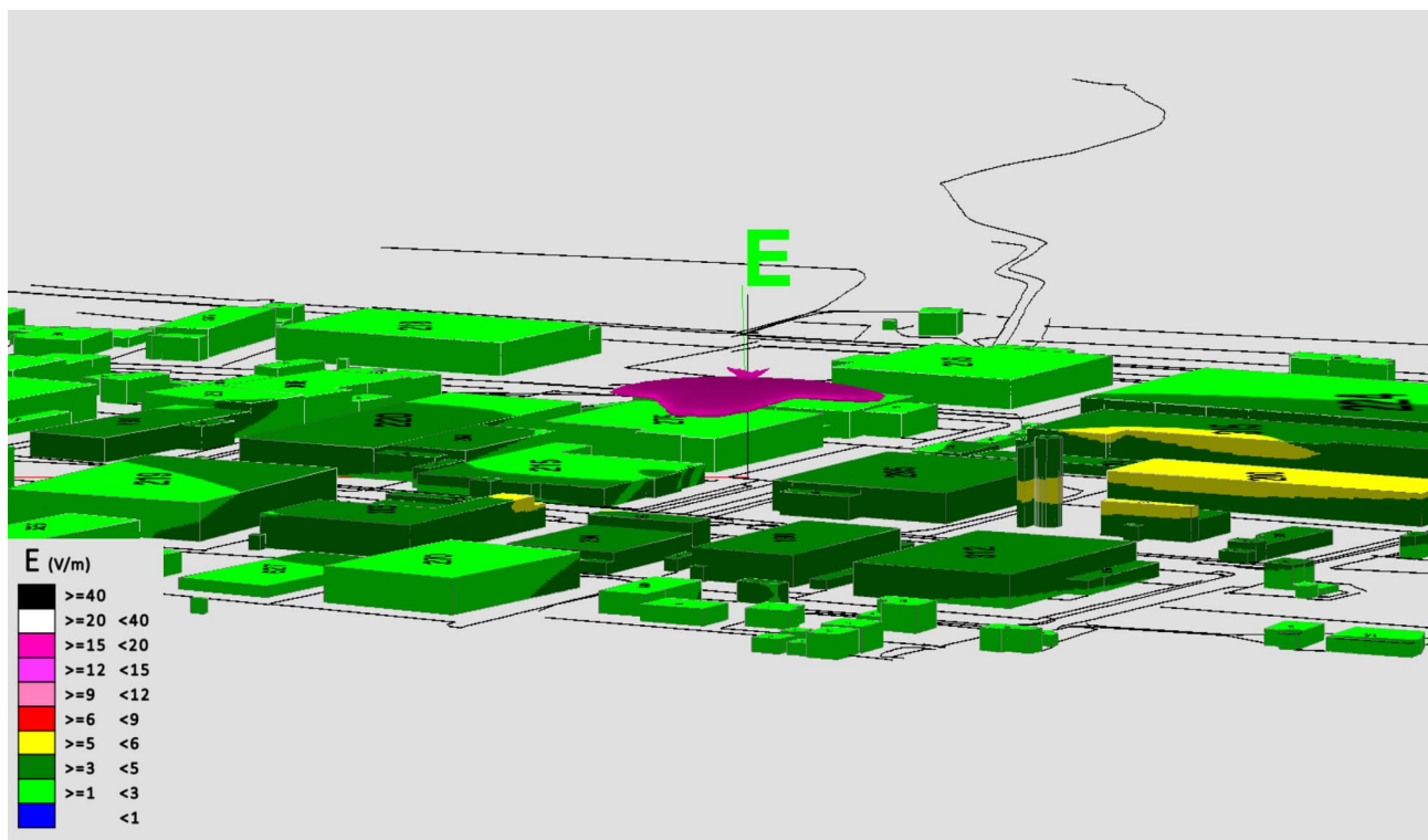
Fig. 29 Impatto elettromagnetico - Zona Area Comunale Via Galileo Galilei - Vista Laterale 1
