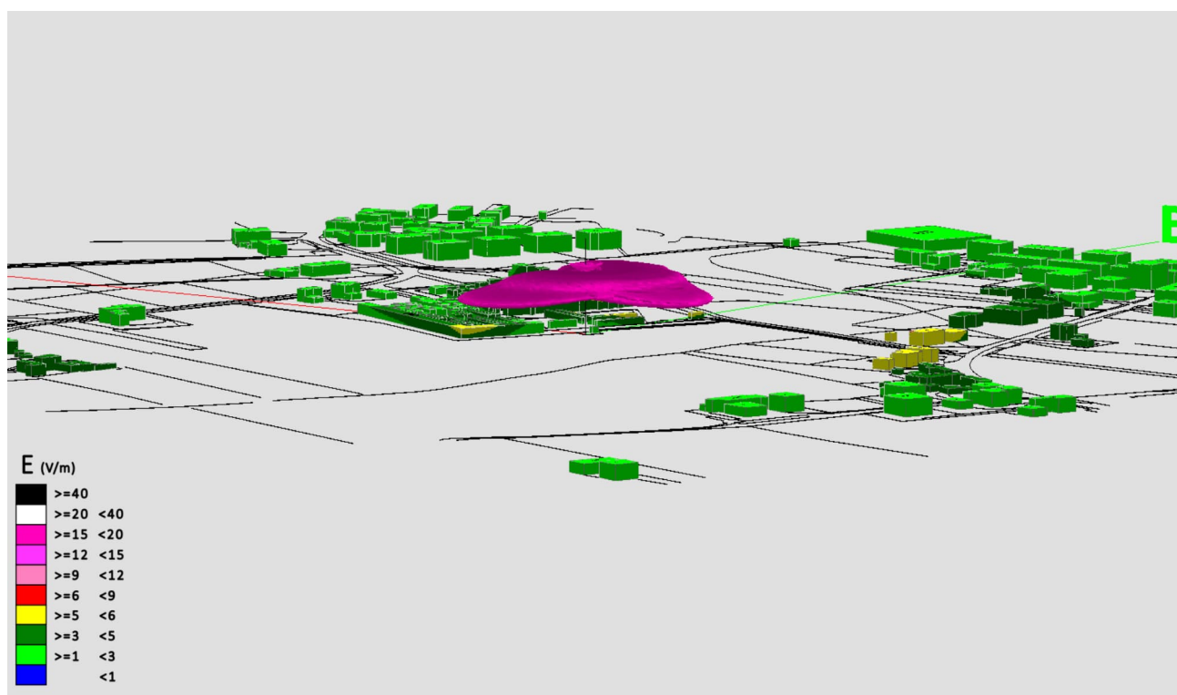
Fig. 9 Impatto elettromagnetico - Zona Cimitero Piove di Sacco 1 - Vista Laterale 1
