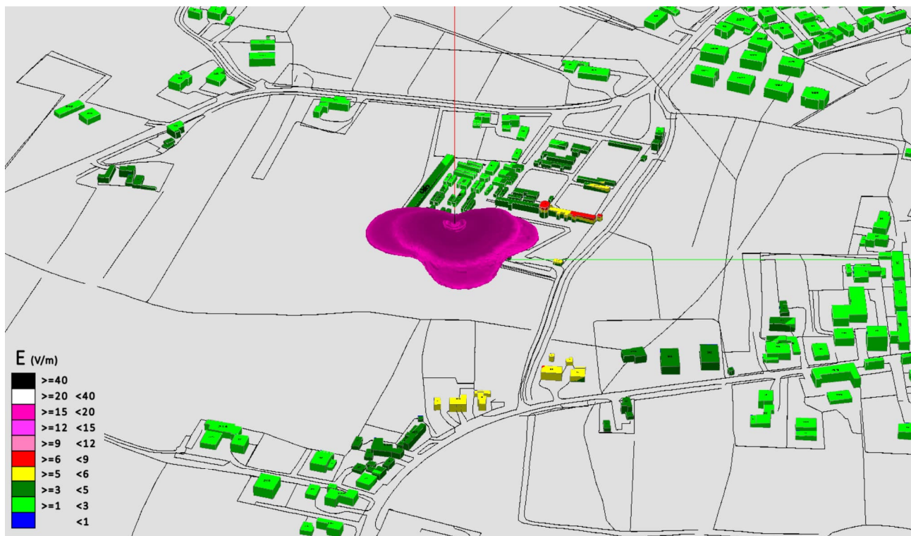
Fig. 7 Impatto elettromagnetico - Zona Cimitero Piove di Sacco 1 - 0°/Nord
