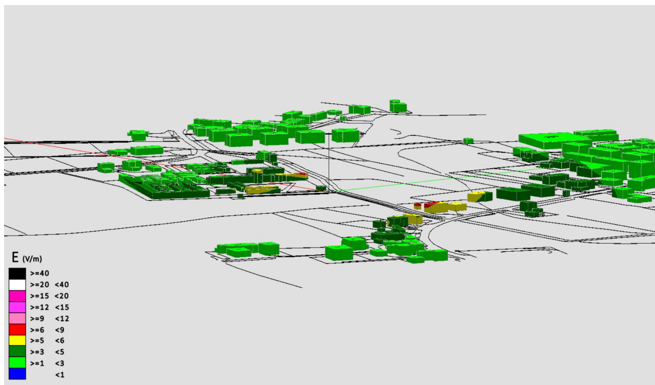
Fig. 15 Impatto elettromagnetico - Zona Cimitero Piove di Sacco 2 - Vista Laterale 2
