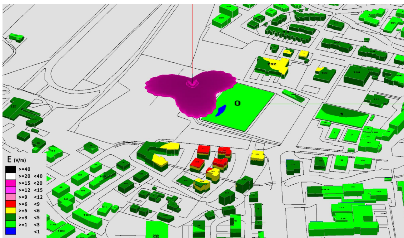
Fig. 2 Impatto elettromagnetico - Zona Area Comunale c/o Stadio - 0°/Nord
