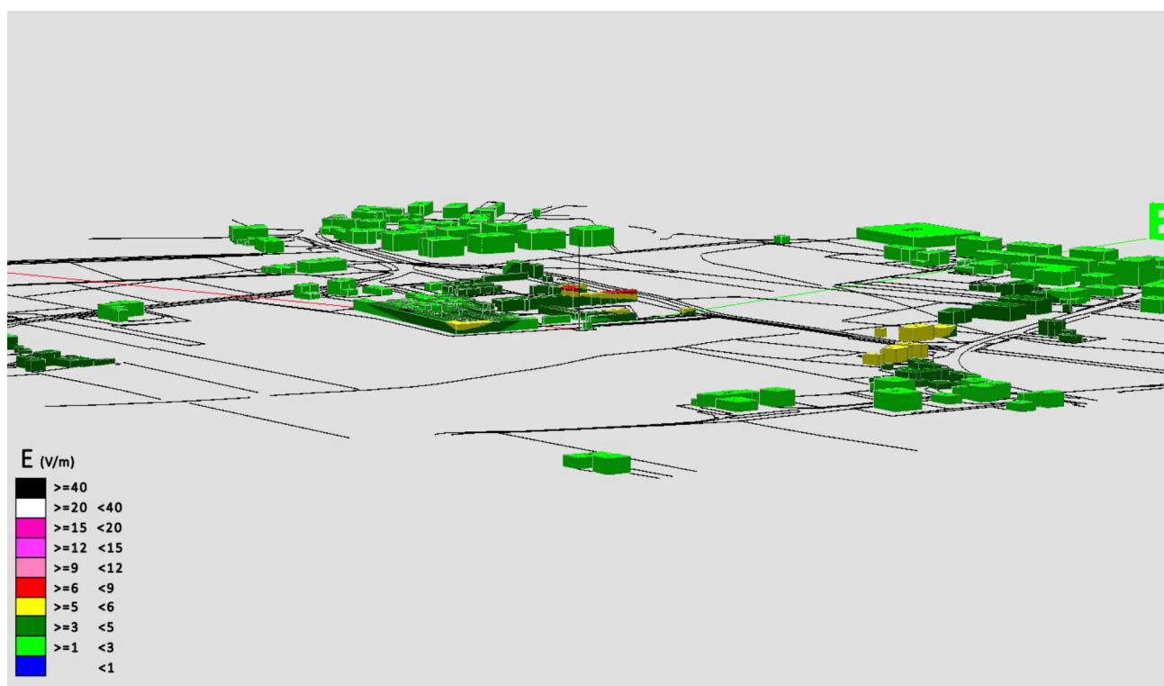
Fig. 10 Impatto elettromagnetico - Zona Cimitero Piove di Sacco 1 - Vista Laterale 2
