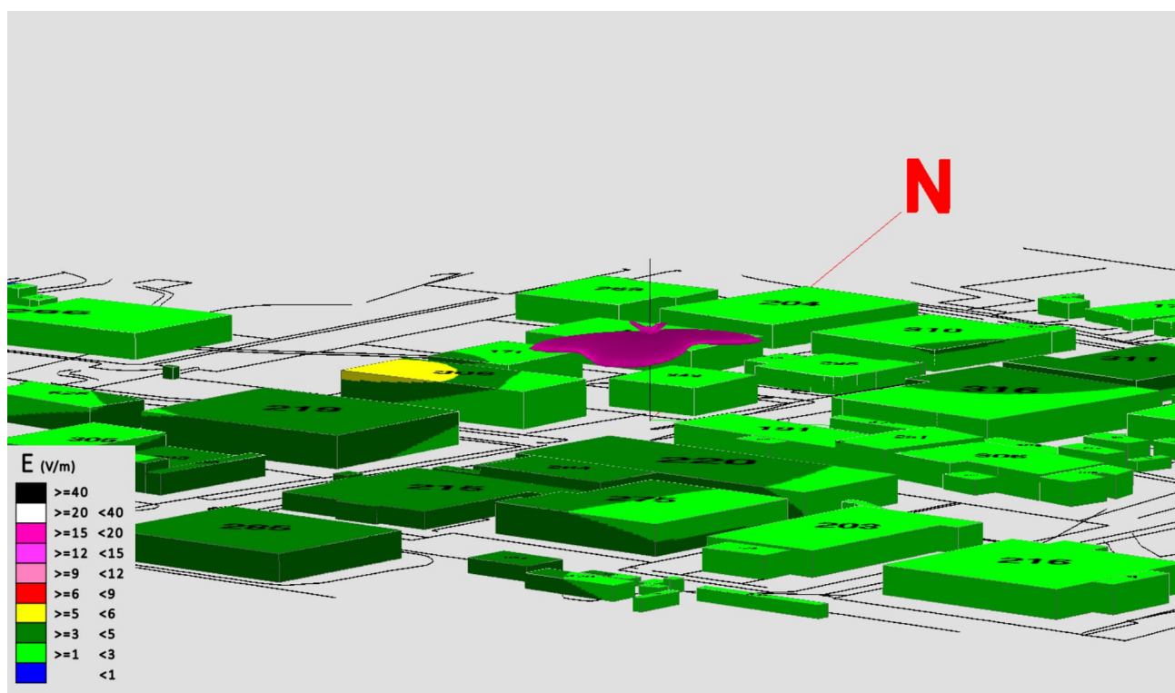
Fig. 34 Impatto elettromagnetico - Zona Area Comunale Via dell'Industria - Vista Laterale 1
