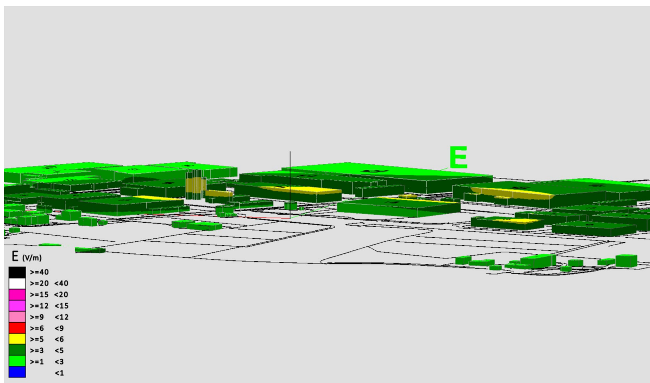
Fig. 20 Impatto elettromagnetico - Zona Area Comunale Via Keplero Nord - Vista Laterale 2
