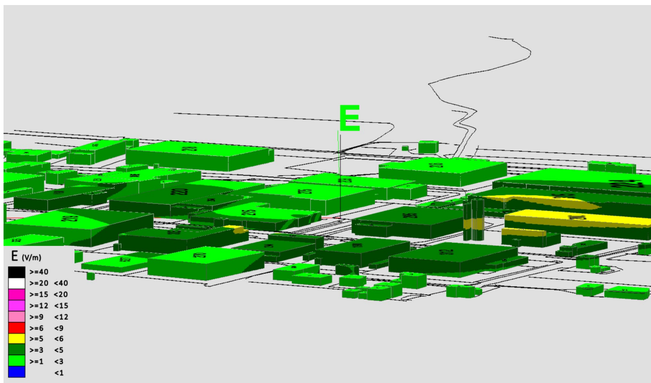
Fig. 30 Impatto elettromagnetico - Zona Area Comunale Via Galileo Galilei - Vista Laterale 2
