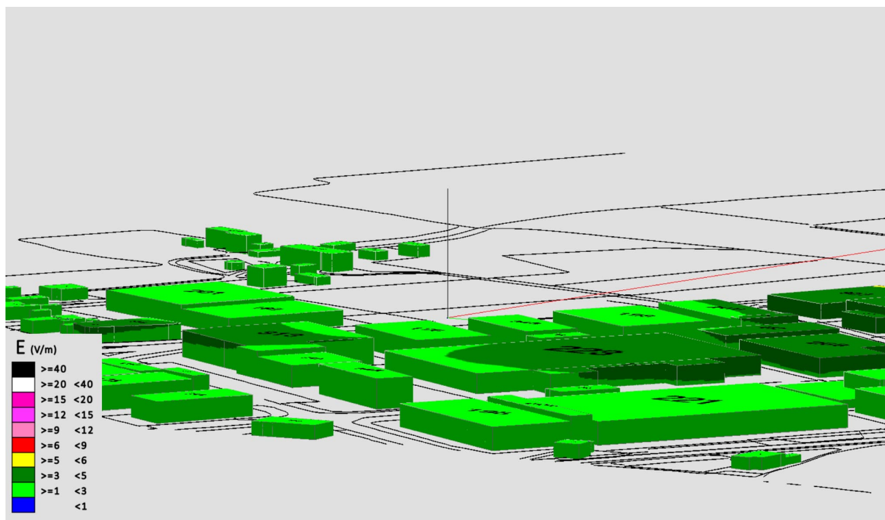
Fig. 25 Impatto elettromagnetico - Zona Area Comunale Via Keplero Sud - Vista Laterale 2
