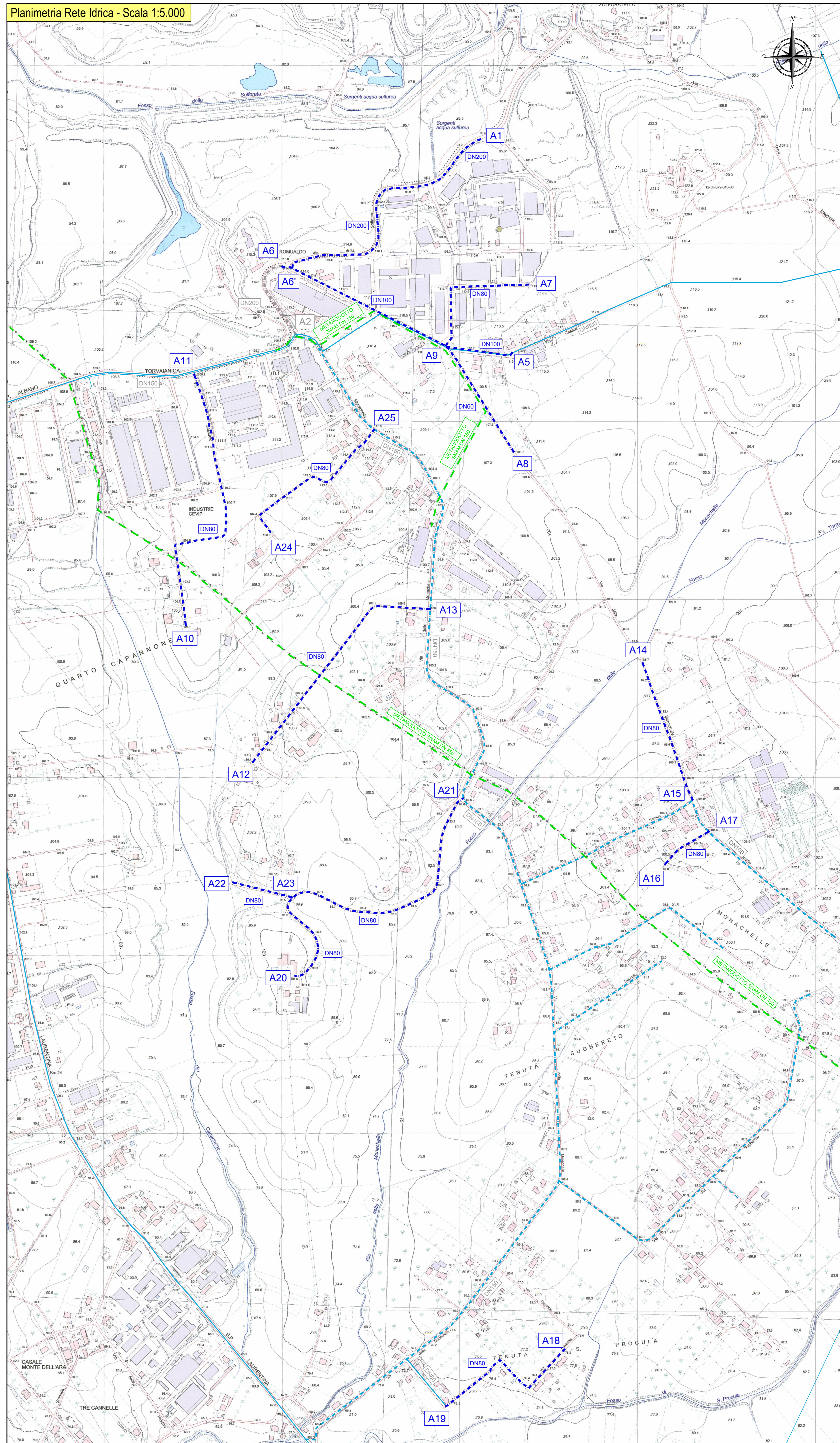
Planimetria Rete Idrica - Scala 1:5.000
