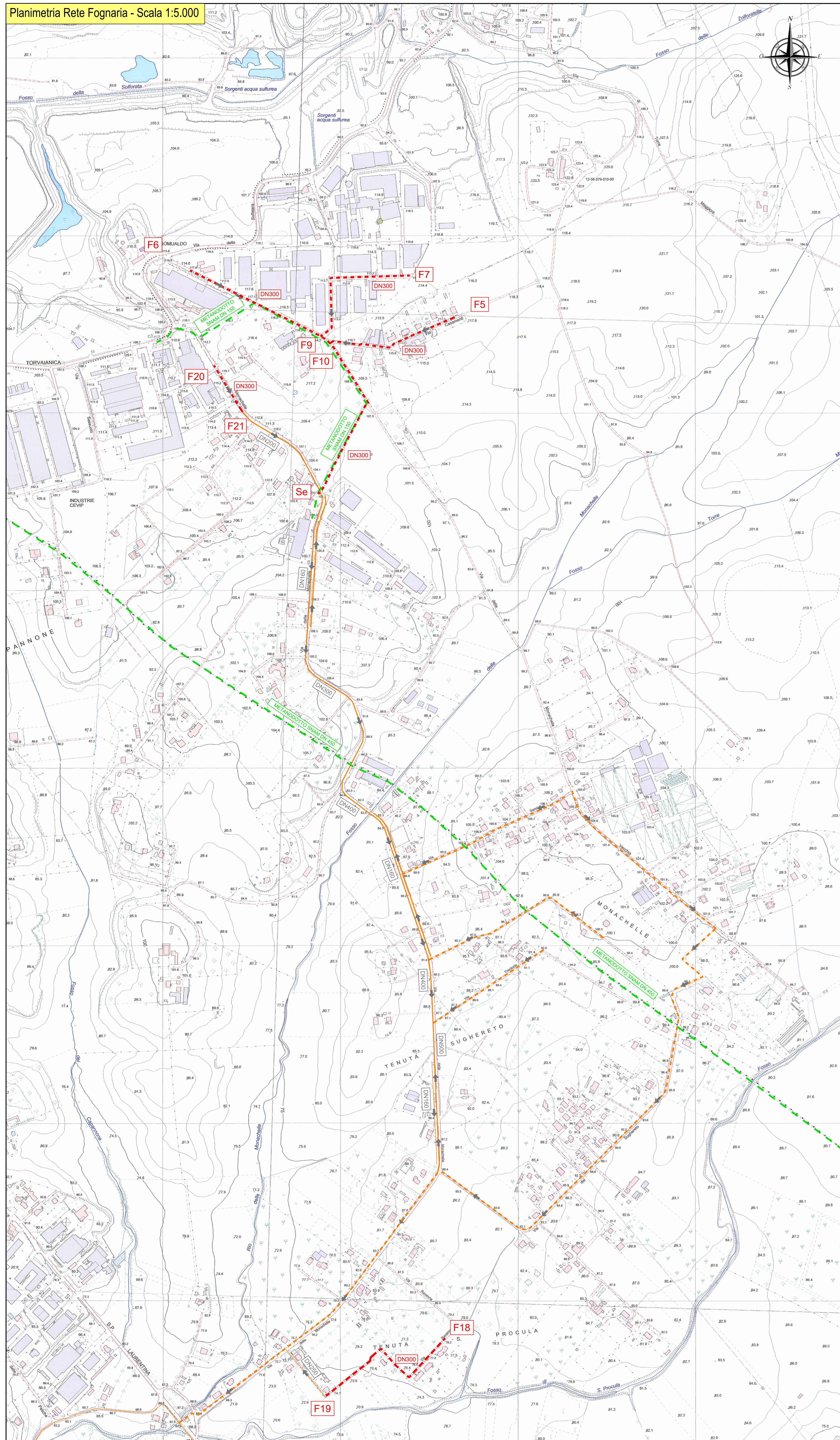
Planimetria Rete Fognaria - Scala 1:5.000
