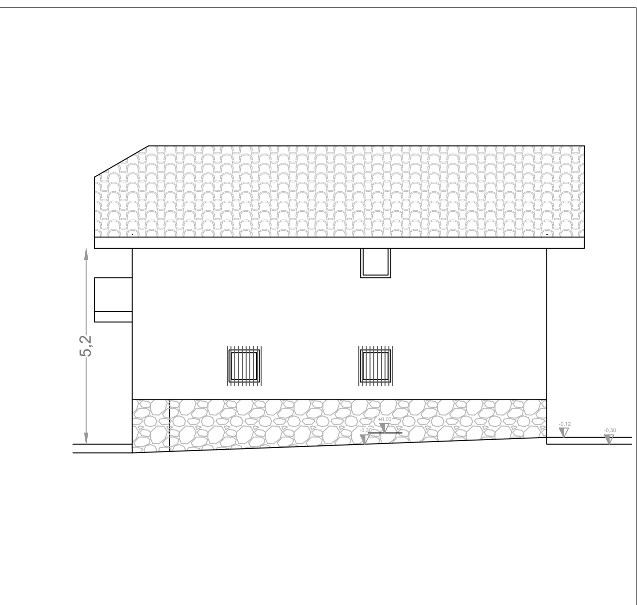
PROSPETTO LATERALE (NORD-OVEST)
