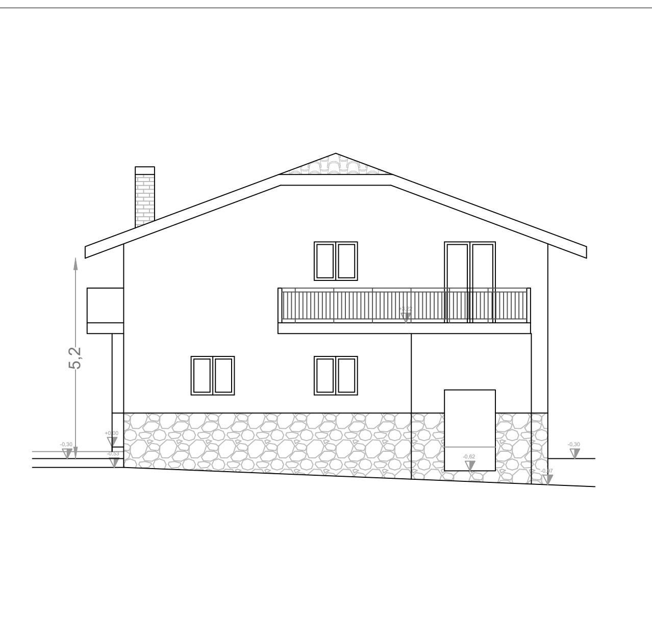
PROSPETTO PRINCIPALE (NORD-EST)
