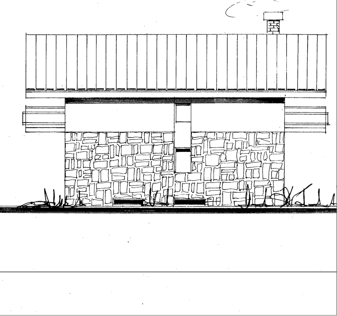
PROSPETTO LATERALE (NORD-OVEST)
