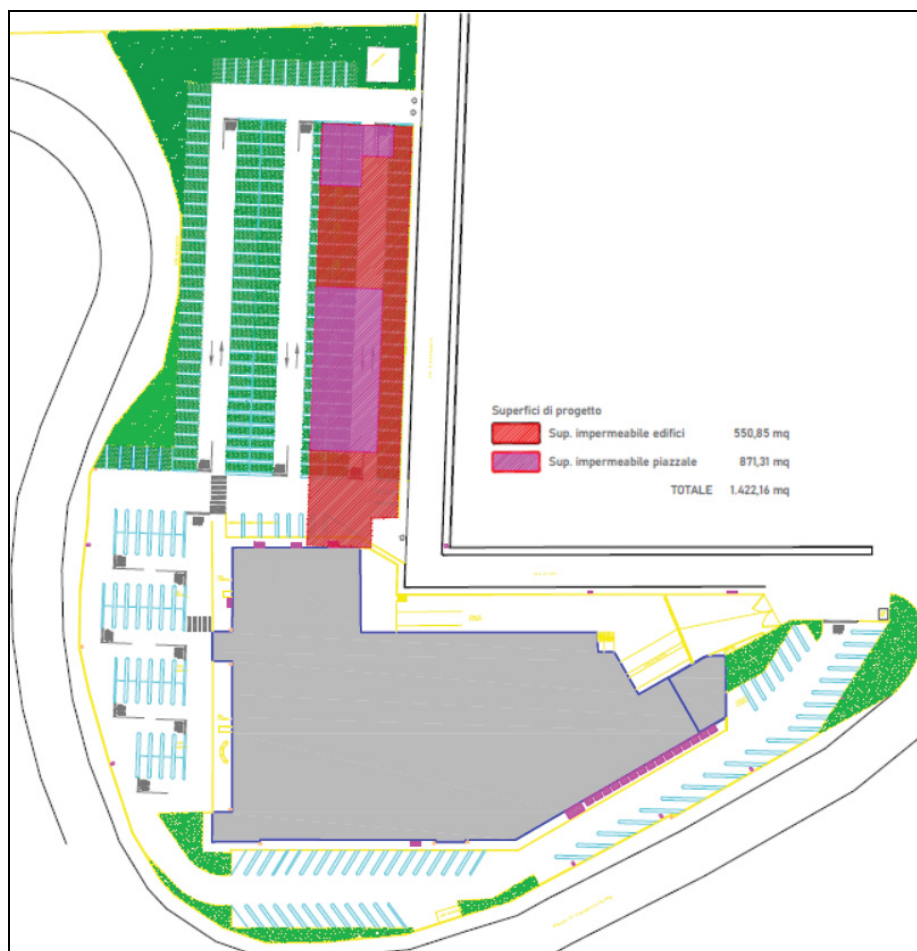
Identificazione delle superfici scolanti del lotto oggetto di misure di invarianza
