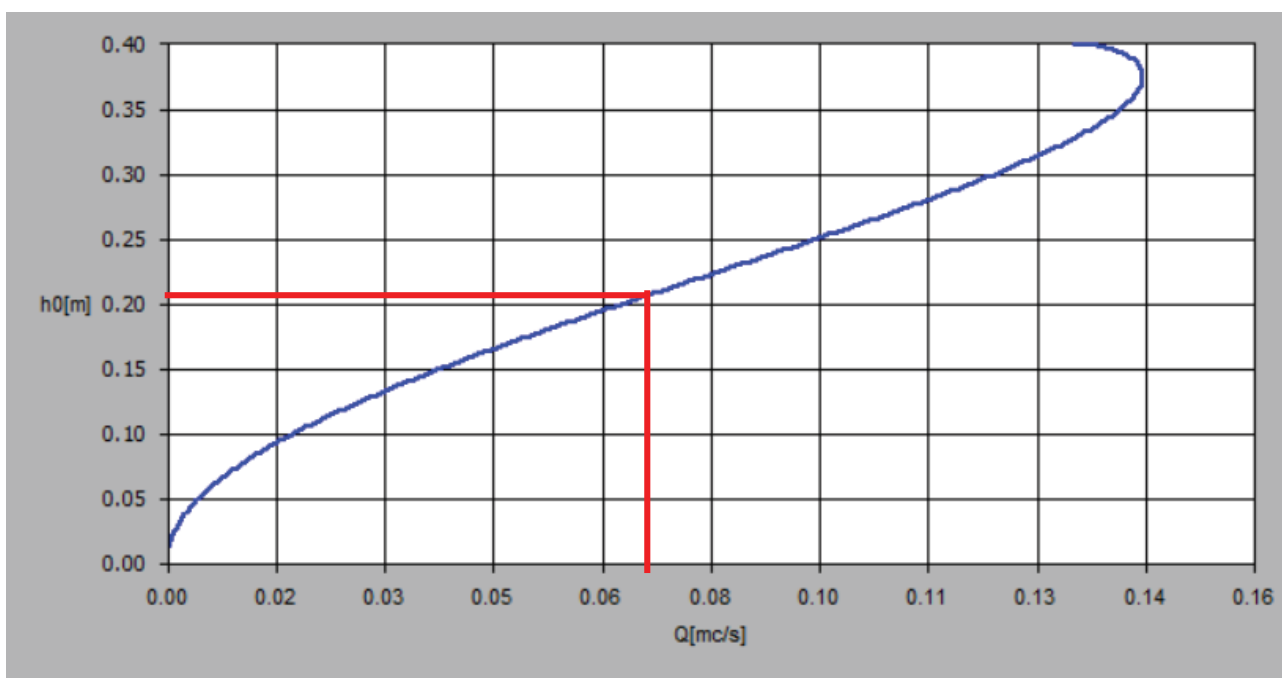
Output di verifica idraulica del collettore in ingresso al sistema
