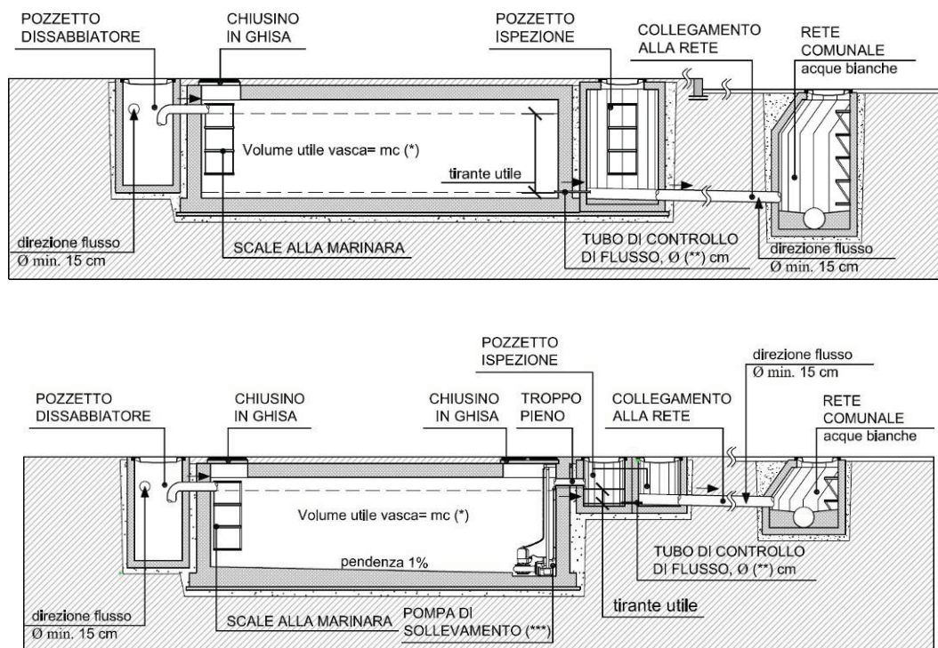
Particolari vasca di laminazione con scarico a gravità (sopra) e con scarico mediante pompaggio (sotto)
